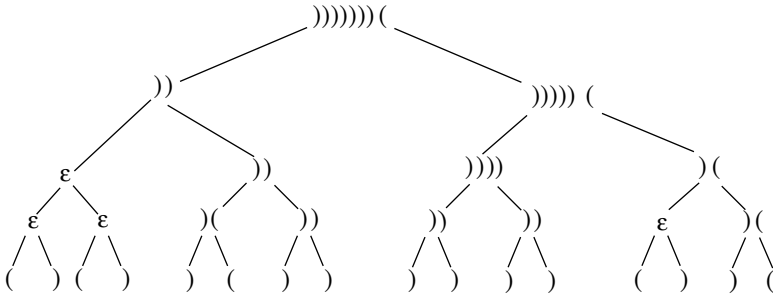
Exemple : arbre réduit de \omega_0 = (00)000000)0(
