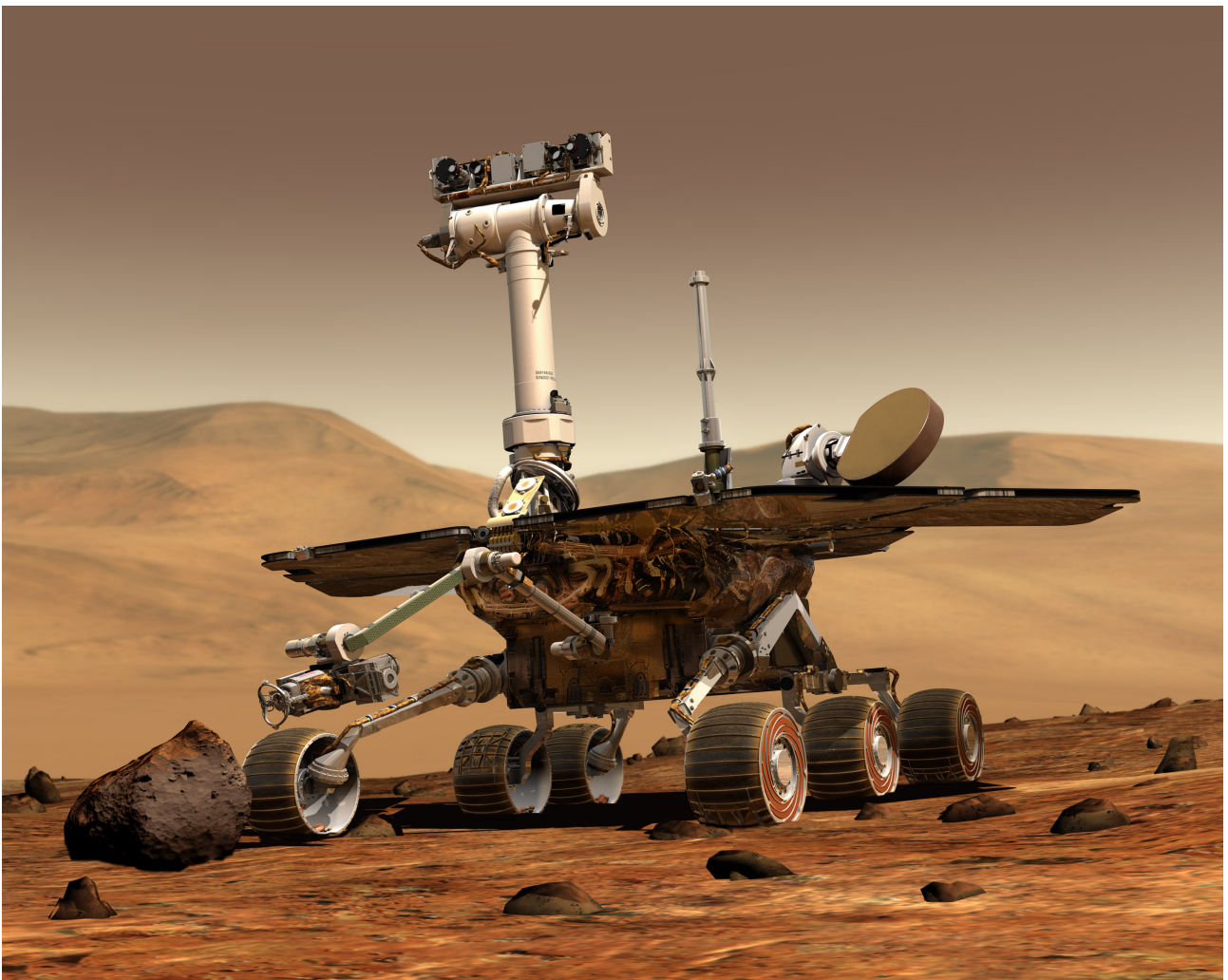
Figure 1 Vue d'artiste d'un robot géologue de la mission Mars Exploration Rovers (NASA/JPL – Caltech/Cornell)
