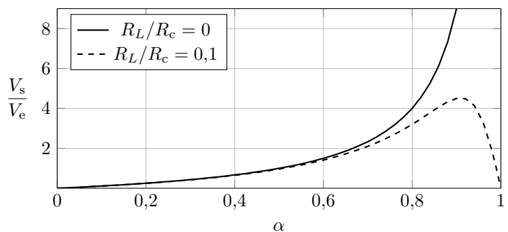
Figure 9 – Gain en fonction du rapport cyclique.
