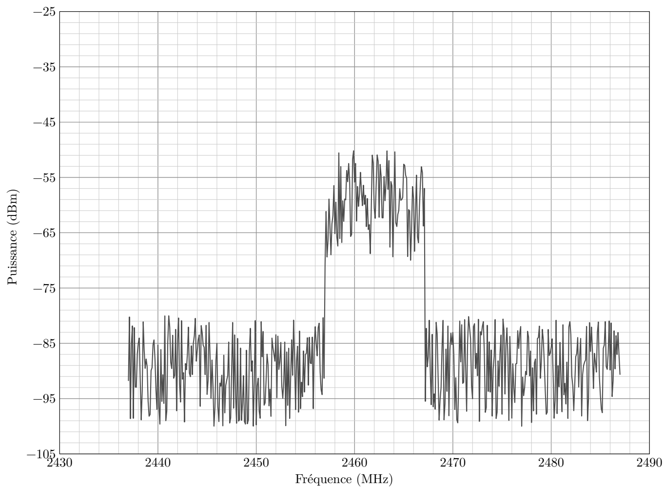
Figure A Relevé spectral de puissance du signal Wi-Fi reçu du Pro-form TDF
