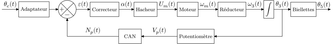
Figure 16 Structure de l'asservissement de position des biellettes
